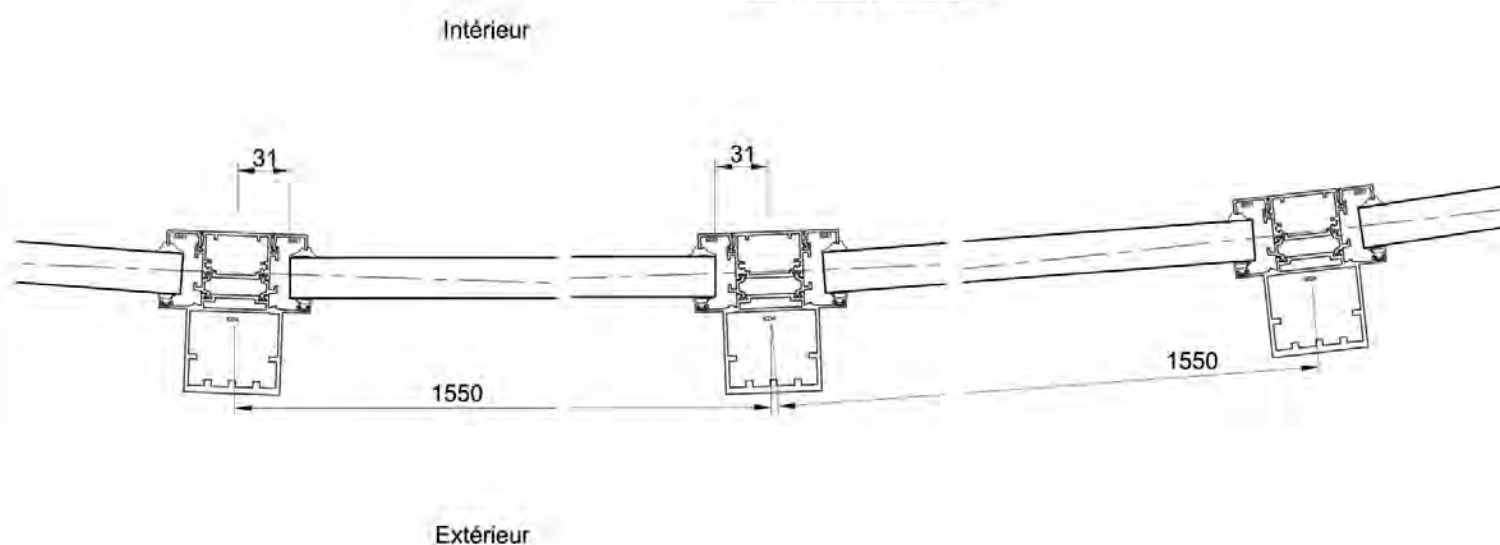
- Coupe A-A (éch. : 1/4) -
