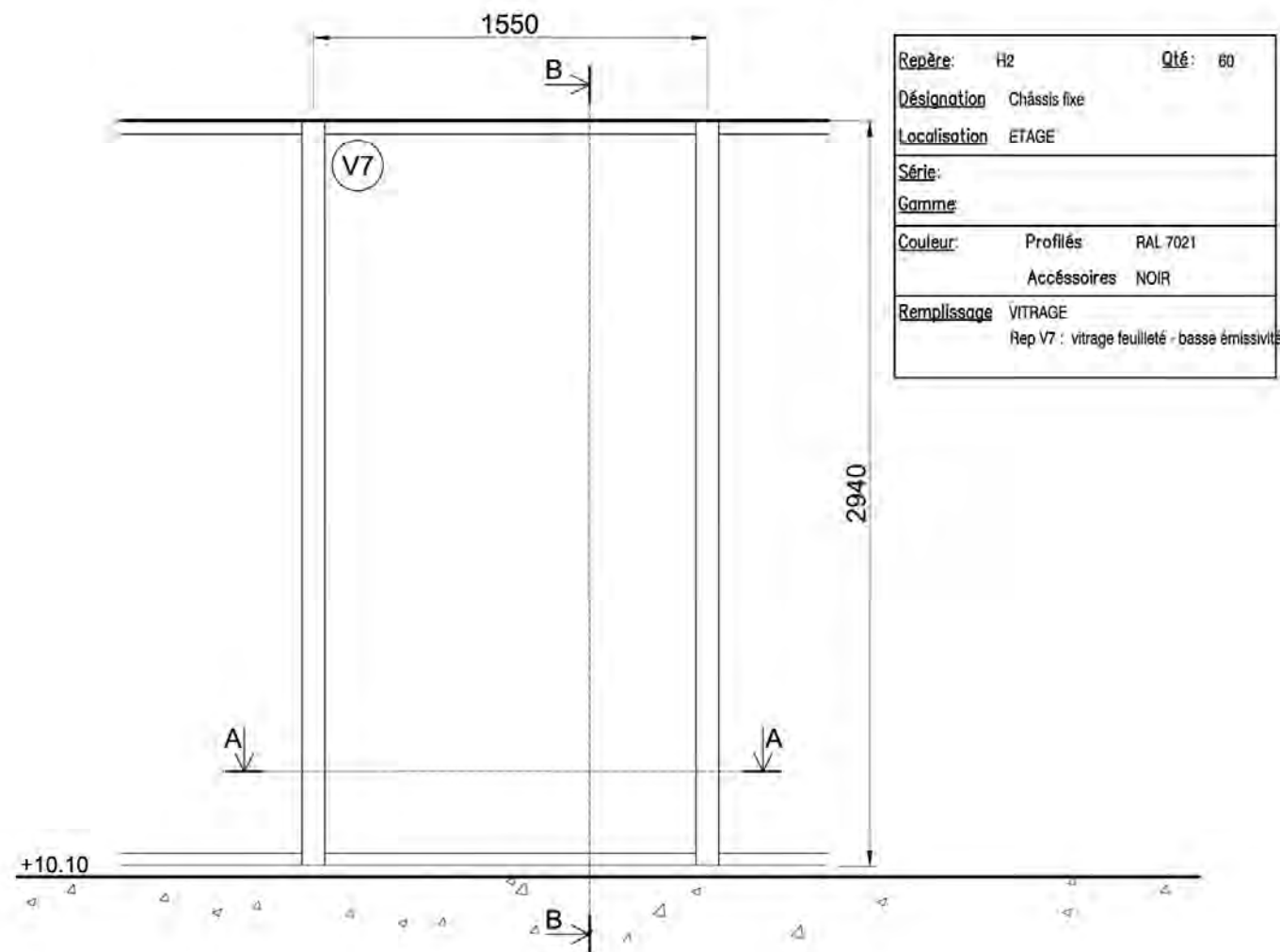
- Elevation vue exterieure (éch. : 1/25) -
