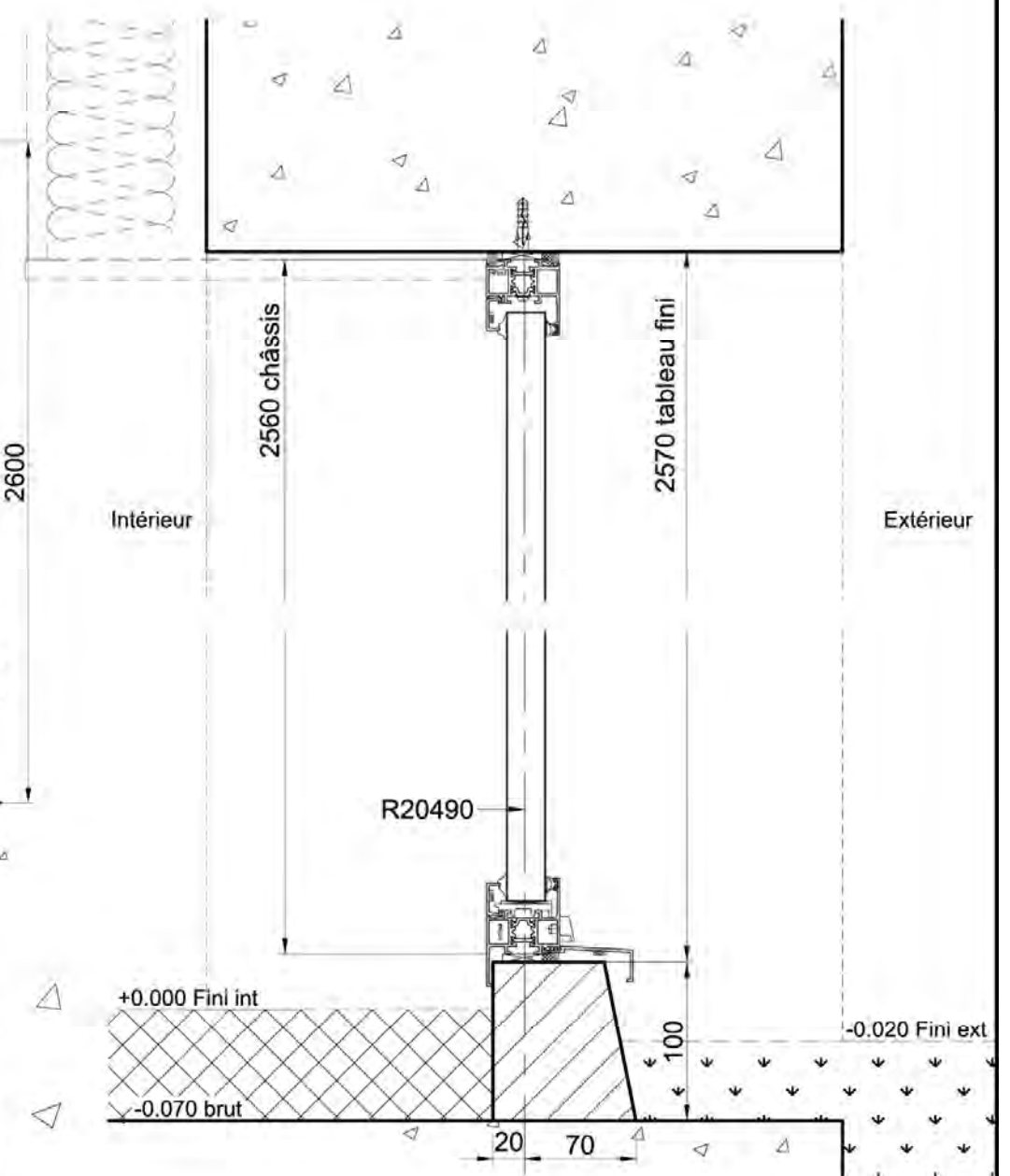
- Coupe B-B (éch. : 1/4) -
