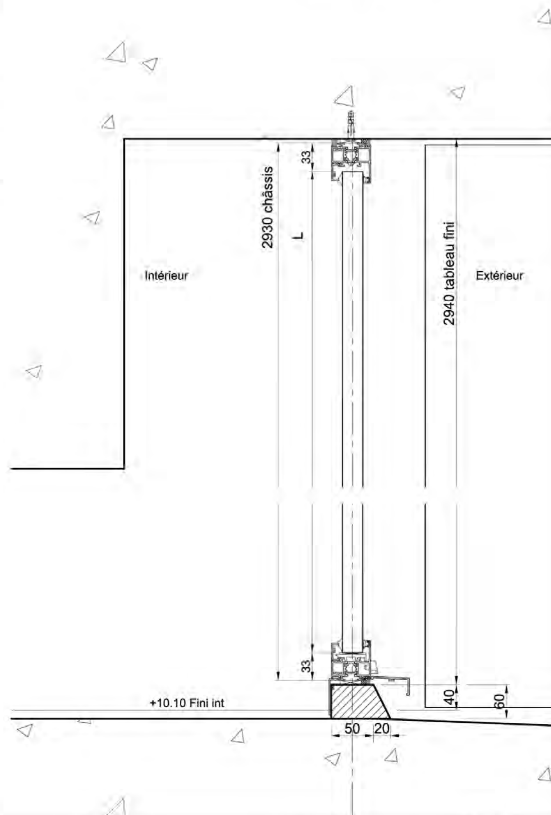
- Coupe B-B (éch. : 1/4) -
