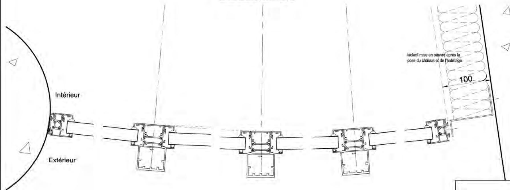
- Coupe A-A (éch. : 1/4) -
